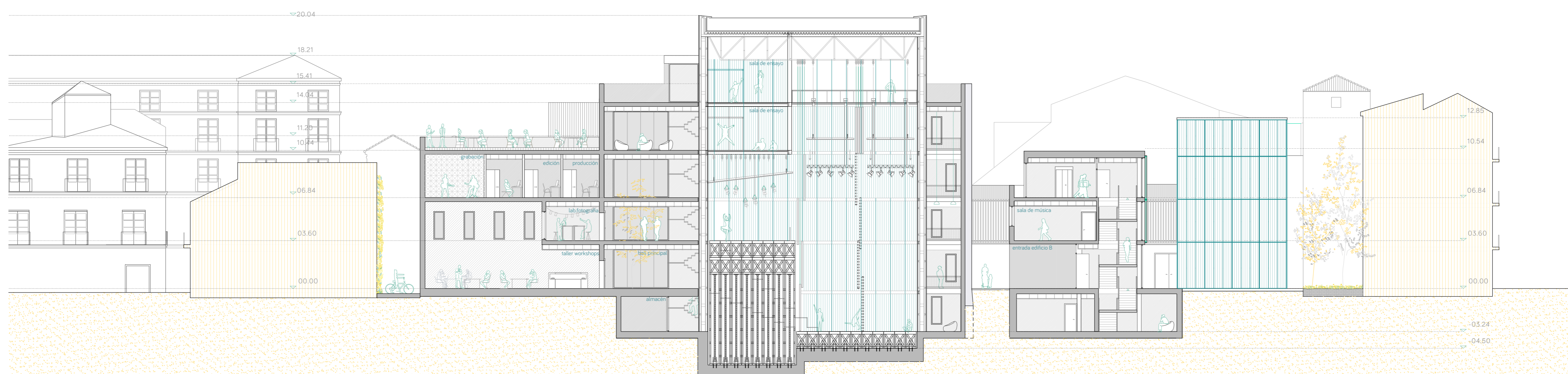
SECCIÓN H-H' e_1_200
