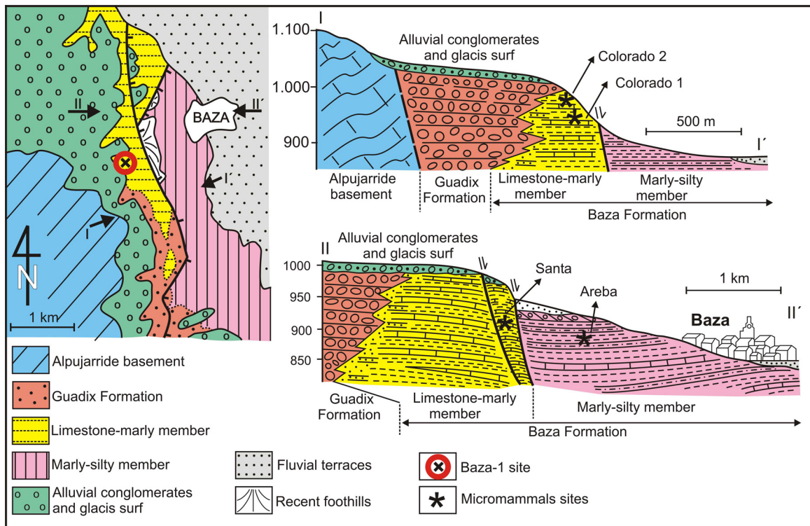
Fig. 2. Geologic map and sections of the Baza area. Fig. 2. Carte géologique et sections de la zone de Baza.
