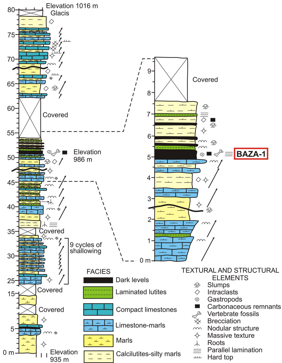
Fig. 3. Stratigraphical column of Baza-1 site. Fig. 3. Colonne stratigraphique du gisement de Baza-1.
