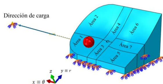
Figura 2. Modelo de EF del espécimen simulado. Fuente: elaboración propia.
