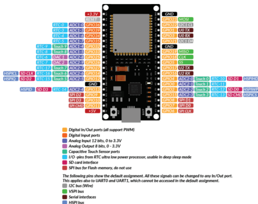
Figura 4.21: Pinout ESP32.
