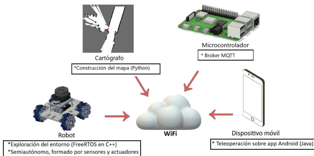
Figura 3.1: Arquitectura básica del sistema.
