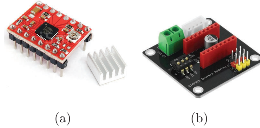
Figura 4.7: A49988 y Módulo de control
