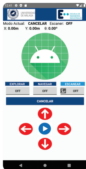
Figura 6.6: Diseño aplicación.
