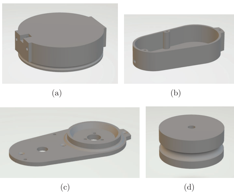
Figura 4.10: Estructura 3D LIDAR escogida.
