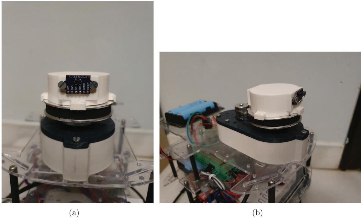
Figura 4.8: LIDAR diseño propio.
