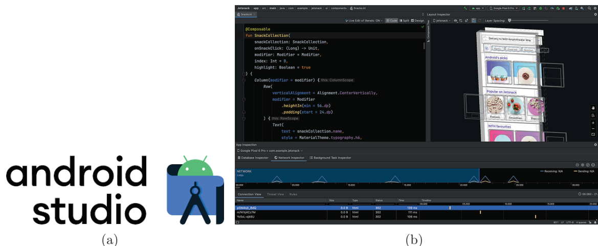
Figura 2.7: Android Studio.
