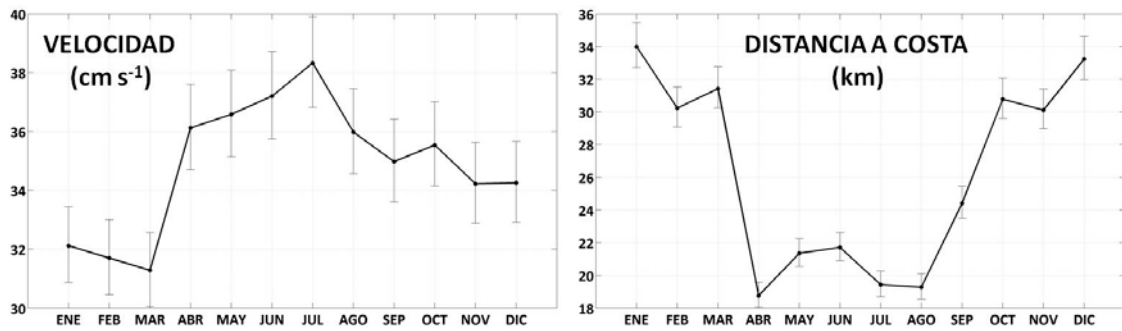
Figura 3.18. Estacionalidad del jet atlántico a su entrada en el mar Alborán a través del estrecho de Gibraltar. La distancia a costa se ha estimado a partir del ángulo del jet en el estrecho de Gibraltar siguiendo a Sarhan et al. (2000). Las barras verticales indican \pm 1 desviación estándar.
