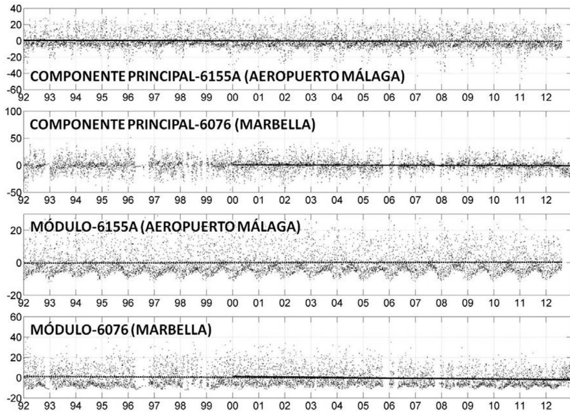
Figura 3.26. Serie temporal de anomalías y de la velocidad del viento en las estaciones del aeropuerto de Málaga y de Marbella ( m s^{-1} ). Las líneas indican las tendencias temporales que fueron significativas estadísticamente. Los resultados completos del análisis se muestran en la Tabla 8.25. (Anexo I).
