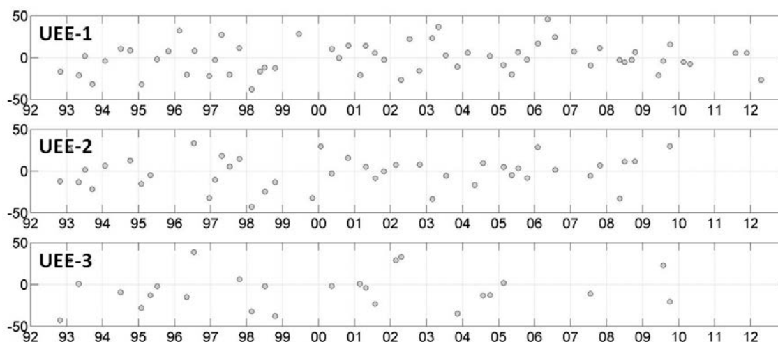
Figura 3.23. Serie temporal de anomalías de la profundidad de la IAM (m). Los resultados completos del análisis se muestran en la Tabla 8.21. (Anexo I).
