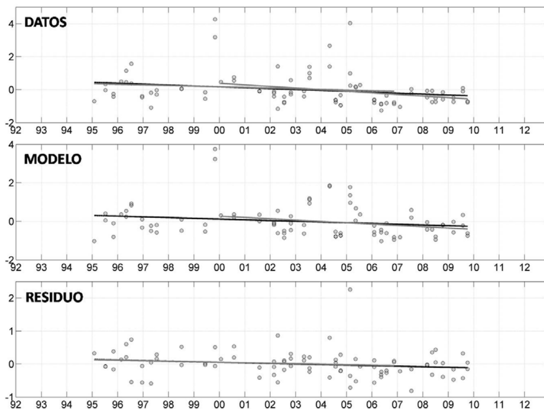
Figura 4.13. Serie temporal de anomalías de los datos observados, del modelo propuesto para UEE-2 y de los residuos ( \text{mg m}^{-3} ). Las líneas continuas indican las tendencias que fueron significativas estadísticamente.
