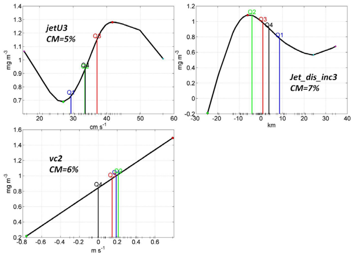
Figura 4.12. Contribución parcial de las variables relacionadas con el jet atlántico y la velocidad zonal de la corriente geostrofica en el modelo propuesto para la UEE-2 en términos de concentración de clorofila.
