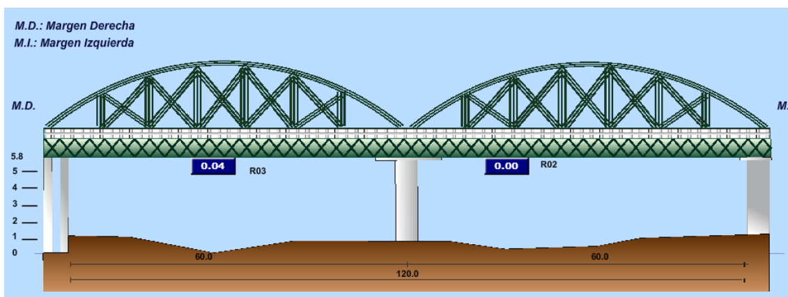
Figura 3.5. Diagrama del cauce del río Guadalhorce en la estación de medida piezométrica de Cártama: ST38 (Fuente: Redhidrosur). Imagen reproducida de http://www.redhidrosurmedioambiente.es .
