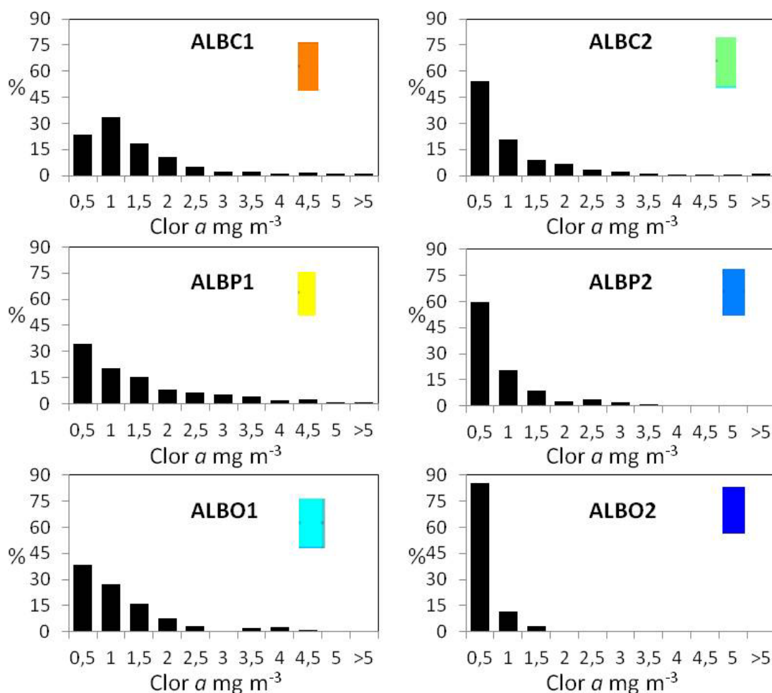
Figura 2.7. Función de distribución por rangos de los valores de concentración de clorofila a para cada clúster. Frecuencia relativa de los valores agrupados en rangos de 0.5 mg m -3 .
