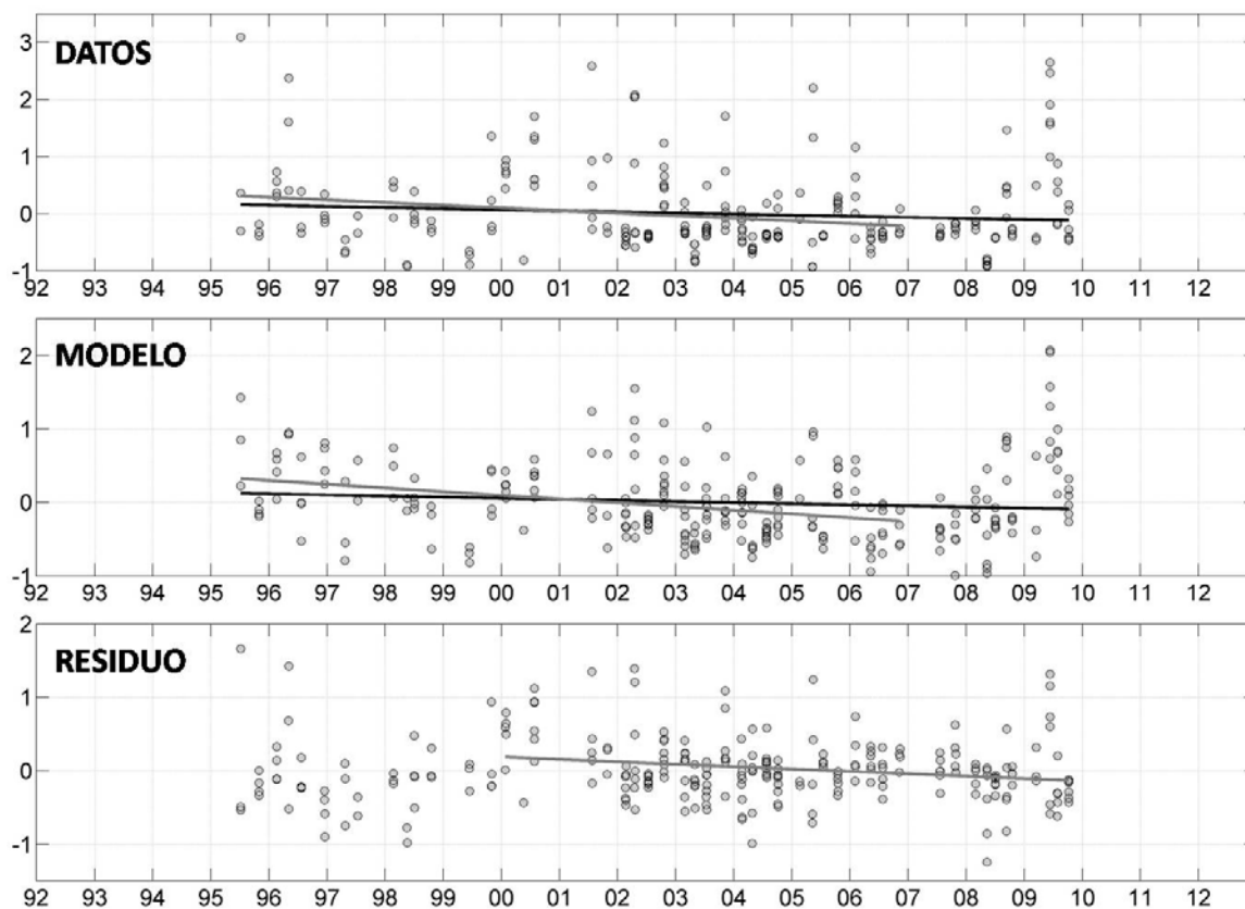
Figura 4.9. Serie temporal de anomalías de los datos observados, del modelo propuesto para UEE-1 y de los residuos ( \text{mg m}^{-3} ). Las líneas continuas indican las tendencias que fueron significativas estadísticamente.
