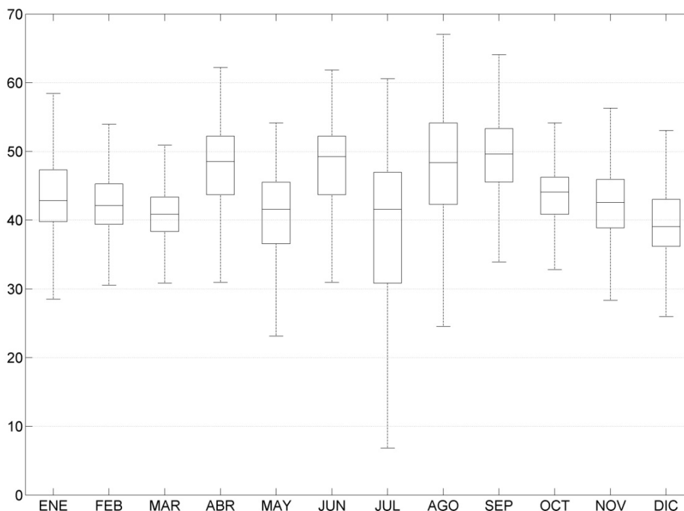
Figura 2.1. Cobertura temporal de los datos de concentración de clorofila-a MODIS-Aqua en el mar Alborán (% de días con datos válidos). Diagrama de Caja o Box-Whisker, donde la línea central representa a la mediana, los límites de la caja son los percentiles 25 y 75, y los dos bigotes representan 1.5 por el recorrido intercuartílico.
