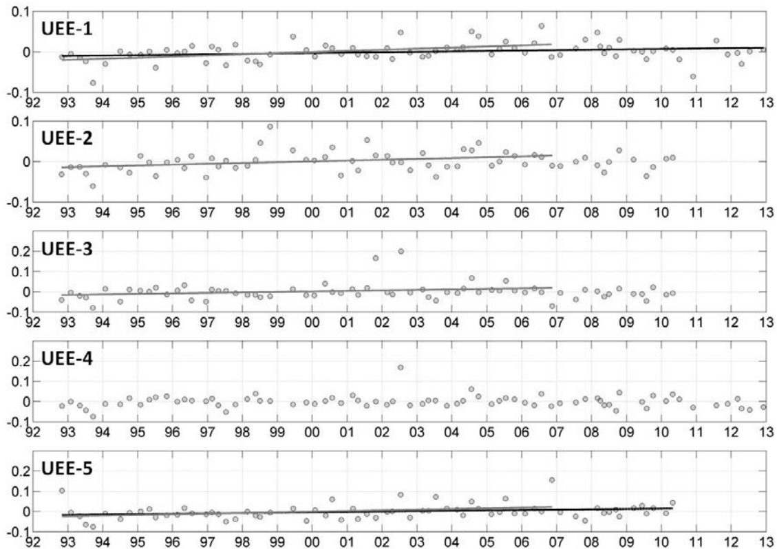
Figura 3.22. Serie temporal de anomalías del SIPIC ( \text{kg m}^{-3} \text{ año}^{-1} ). Las líneas indican las tendencias temporales que fueron significativas estadísticamente. Los resultados completos del análisis se muestran en la Tabla 8.19. (Anexo I).
