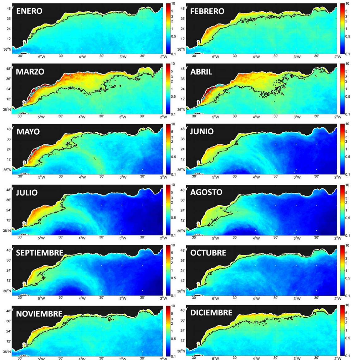
Figura 5.9. Percentil 90 de la concentración de clorofila a calculado para cada mes a partir de los valores obtenidos con el algoritmo ALBOC3 para la serie temporal de 2002 a 2012. La línea negra representa el valor de 1 \text{ mg m}^{-3} , y la cian el valor de 5 \text{ mg m}^{-3} .
