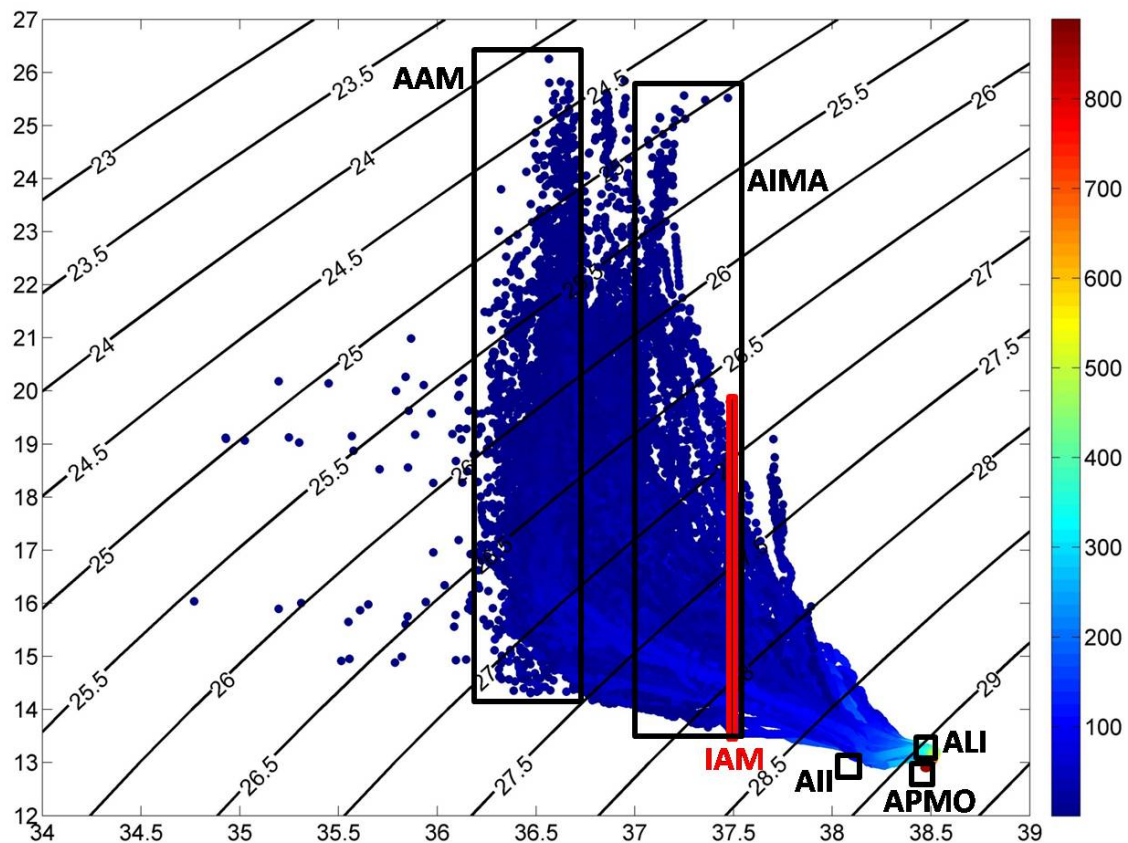
Figura 1.1. Diagrama \theta - S de las masas de agua en la zona noroccidental del mar Alborán (aprox. 1000 perfiles medidos desde 1992 a 2012). La gama de colores expresa la profundidad en metros. Las isolíneas se corresponden con los valores de la densidad de exceso ( \sigma_\theta ). Se han representado rectángulos marcando los valores límite de la Tabla 1.2. Nótese que la AII podría haber desaparecido del norte del mar Alborán en los últimos años (Vargas-Yáñez et al., 2002).
