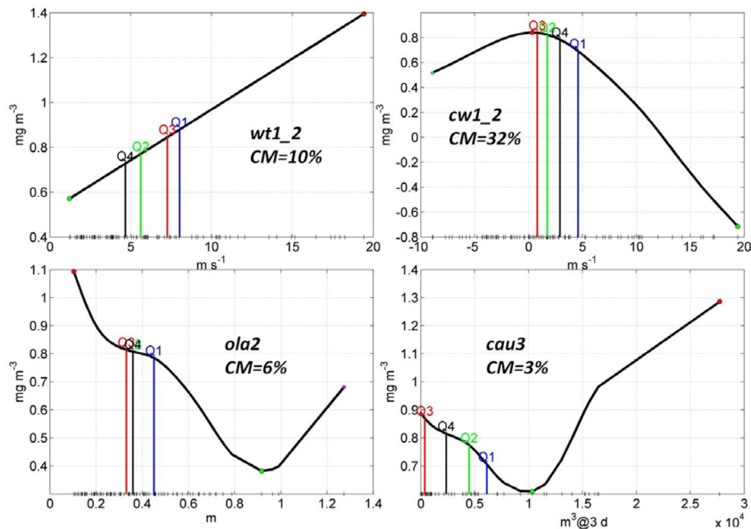
Figura 4.8. Contribución parcial de las variables meteorológicas y ambientales en el modelo propuesto para UEE-1 en términos de concentración de clorofila.
