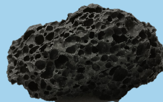
Basalto
