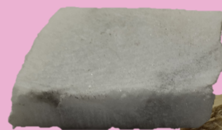
Mármol
