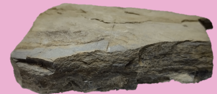
Esquisto
