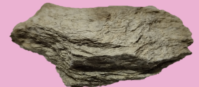
Esquisto
