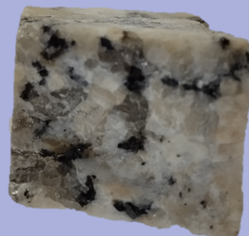
Granito
