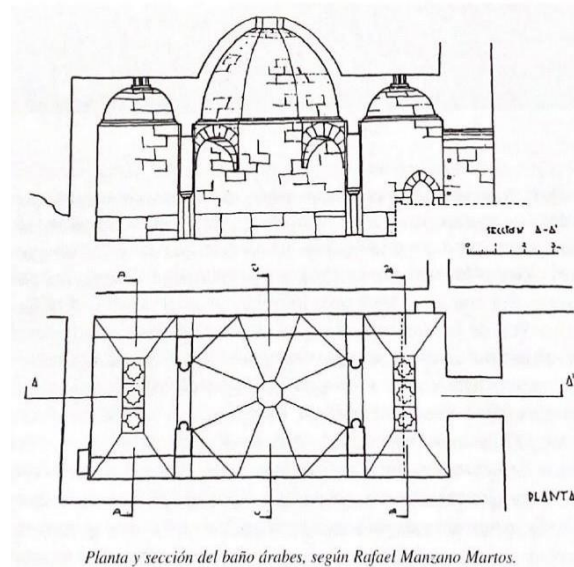
Planta y sección del baño árabes, según Rafael Manzano Martos.
