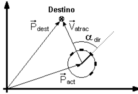
Figura 5.18: Cálculo de la dirección de avance en línea recta el destino final.
