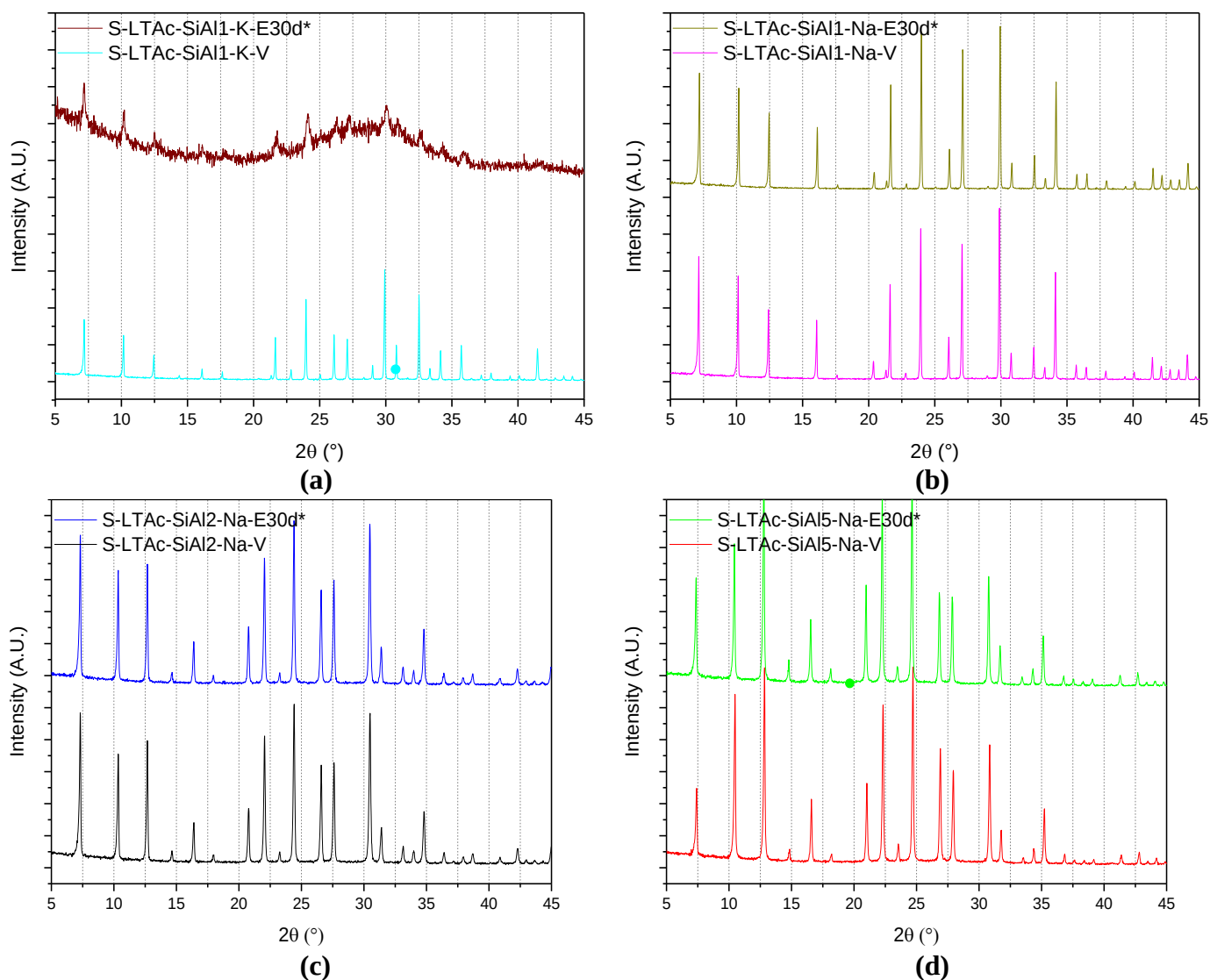
Figure 5.3.1. XRD Diffractograms for S-LTAc-SiAl1-K- (V, E30d*) (a), S-LTAc-SiAl1-Na- (V, E30d*) (b), S-LTAc-SiAl2-Na- (V, E30d*) (c) and S-LTAc-SiAl5-Na- (V, E30d*) (d)
