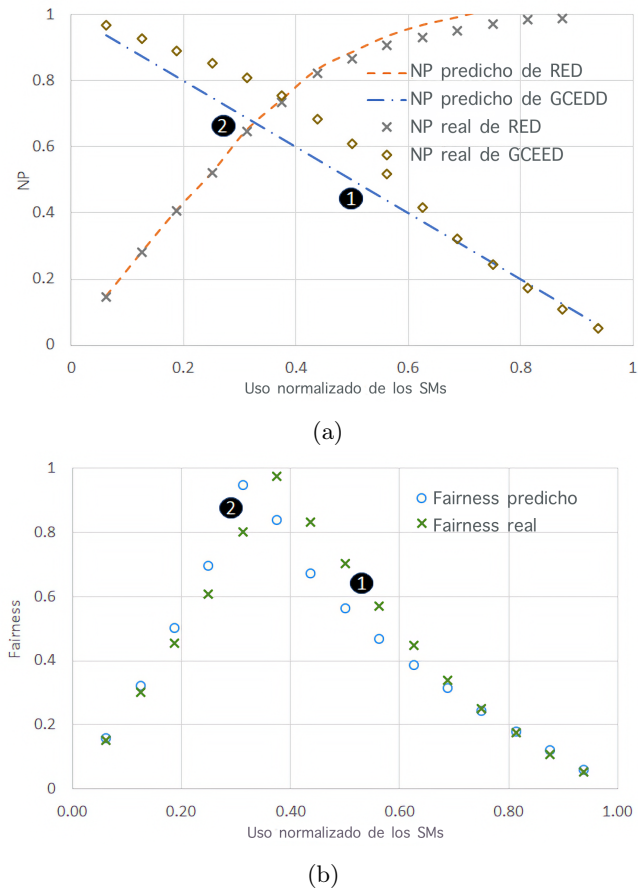
Figura 5.4: (a) NP y (b) Fairness para HSM-Fair aplicado a la coejecución SMK de RED y GCEED
