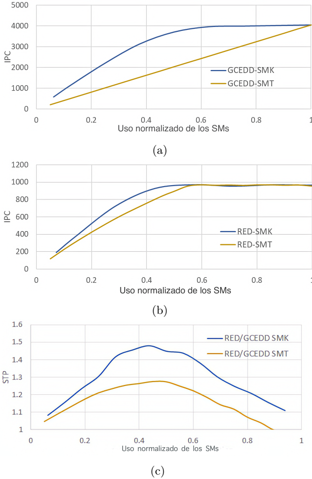
Figura 5.1: IPC alcanzado por la ejecución individual de los kernels (a) GCEDD y (b) RED utilizando un número variable de CTAs mediante SMT y SMK. (c) Rendimiento del sistema ( STP ) obtenido durante la coejecución de los kernels RED y GCEDD para diferentes políticas de planificación de los recursos SMT y SMK.
