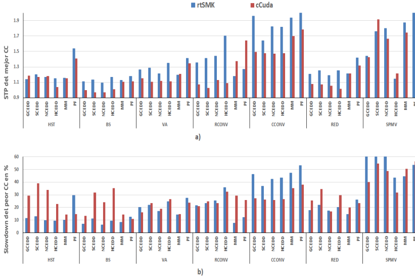
Figura 4.7: FlexSched versus cCUDA. a) muestra los STP máximos alcanzados por el mejor CC cuando se coejecutan los pares de kernels CB y MB utilizando nuestro esquema de planificación de CTAs ( rtSMK ) y el esquema de slicing de cCUDA. Se puede observar que nuestra técnica es capaz de obtener mejores resultados en la mayoría de casos. Así, el STP medio obtenido por rtSMK es de 1,40 mientras que el STP de cCUDA solo consigue 1,29. b) muestra el slowdown respecto al mejor STP cuando se utiliza la configuración CC que obtiene el menor STP . El slowdown medio de ambos métodos se sitúa en torno al 29 %, lo que indica que la selección de un buen CC es primordial para obtener un buen rendimiento.
