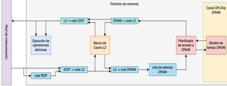
Figura 2.15: Partición de memoria en GPGPU-Sim.
