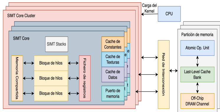
Figura 2.13: Arquitectura GPGPU-Sim.
