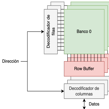
Figura 5.2: Memoria DRAM. Cada banco de memoria posee su decodificador de fila, su row buffer y su decodificador de columna. Con la fila seleccionada y la columna, se accede al dato buscado.
