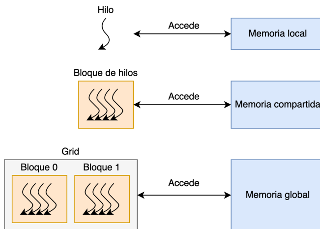
Figura 2.12: Jerarquía de acceso a memoria en CUDA.
