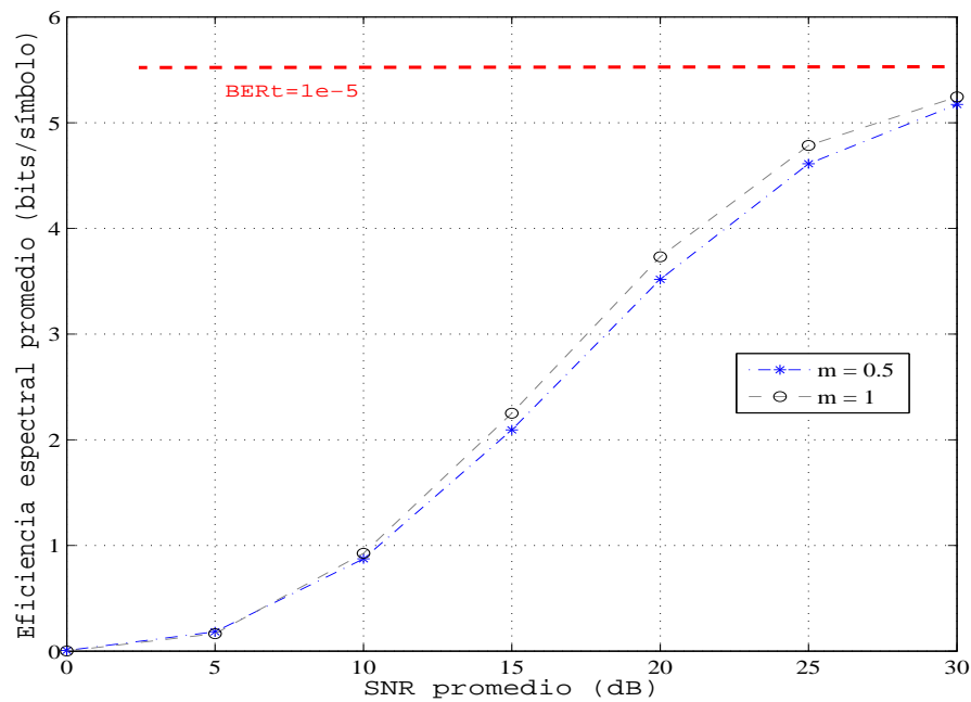
Figura 3.10: ASE vs. SNR promedio para simulaciones de un canal tipo RS con los valores de los parámetros m = 0.5 , 1 y \kappa = 3 dB, usando codificación trellis 4D y \text{BER}_t = 10^{-5} .
