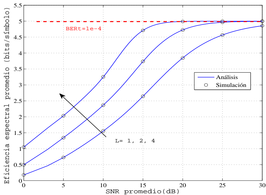
Figura 4.4: ASE vs. SNR promedio para canales independientes tipo RS con los valores de los parámetros m = 1 y \kappa = 10 dB, usando codificación turbo y BER_t = 10^{-4} .
