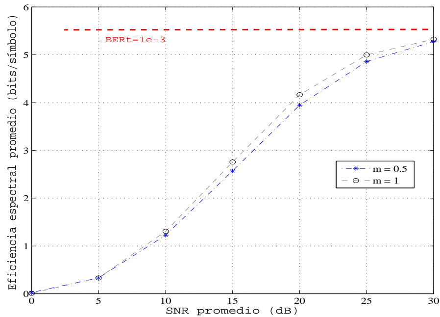
Figura 3.9: ASE vs. SNR promedio para simulaciones de un canal tipo RS con los valores de los parámetros m = 0.5 , 1 y \kappa = 3 dB, usando codificación trellis 4D y \text{BER}_t = 10^{-3} .
