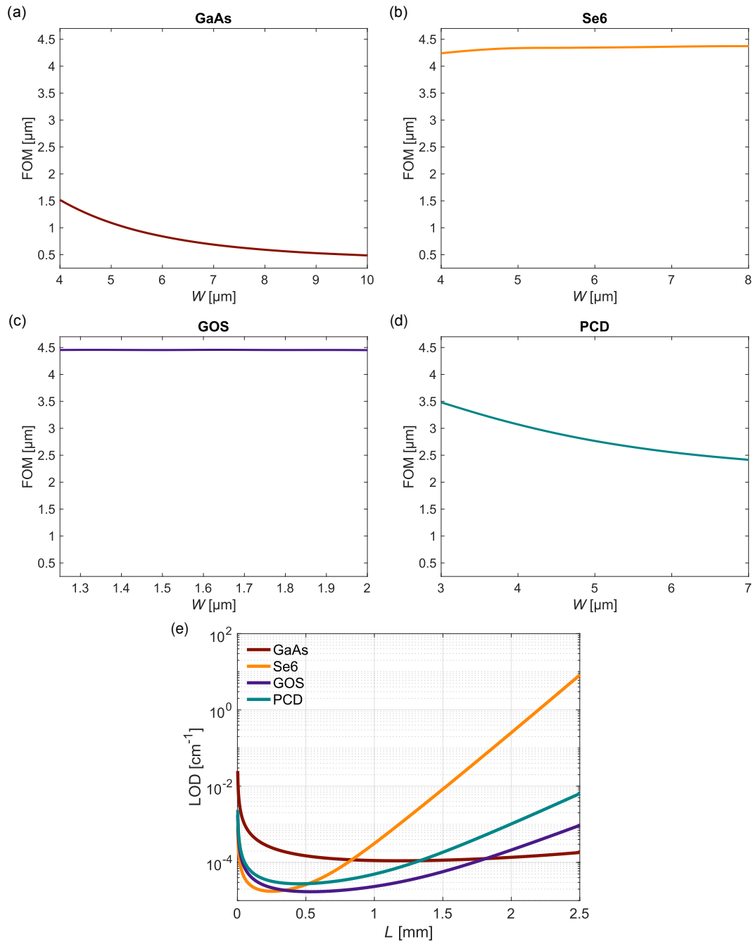
Figura G.19: Figura de mérito de las guías de (a) GaAs, (b) Se6, (c) GOS y (d) PCD waveguides, evaluada en el régimen monomodo. (e) Estimación del límite de detección de cada plataforma.
