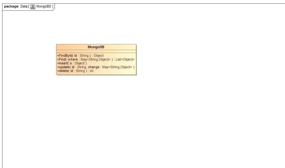
Ilustración 4 Clase MongoDB
