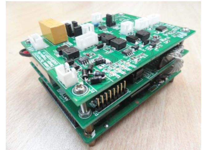
Fig. 40. Modem prototype.
