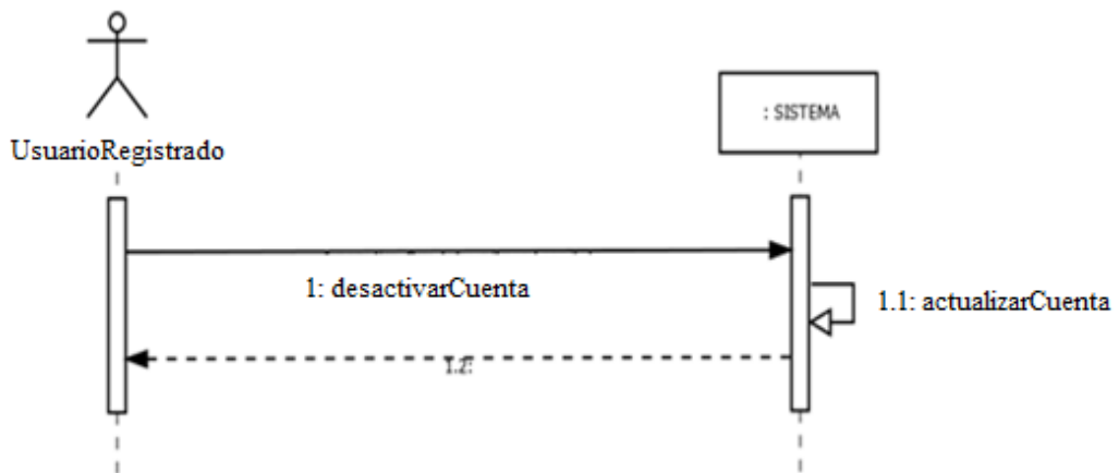
Figura 8. Esquema de la desactivación de la cuenta.
