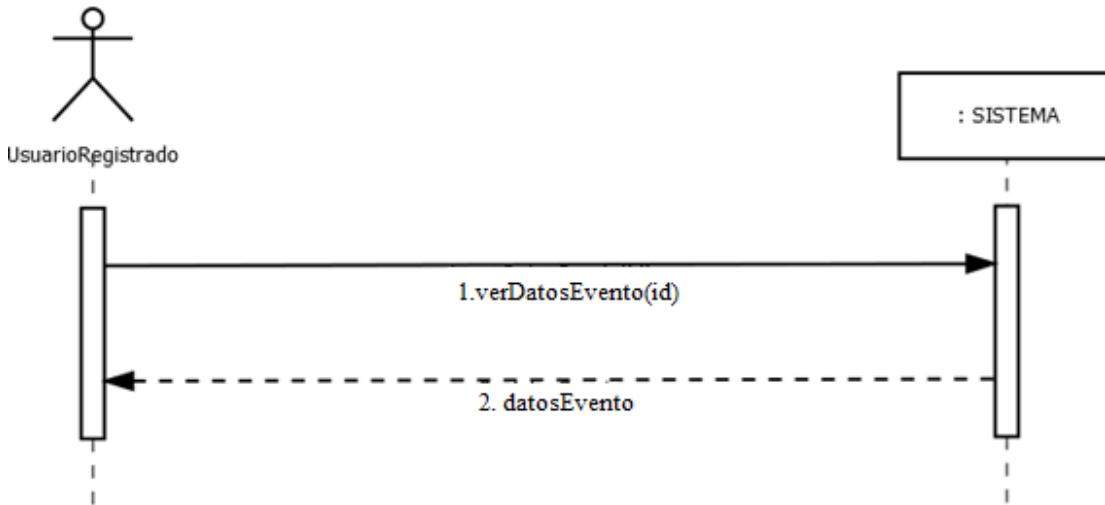
Figura 11. Esquema ver datos del evento.
