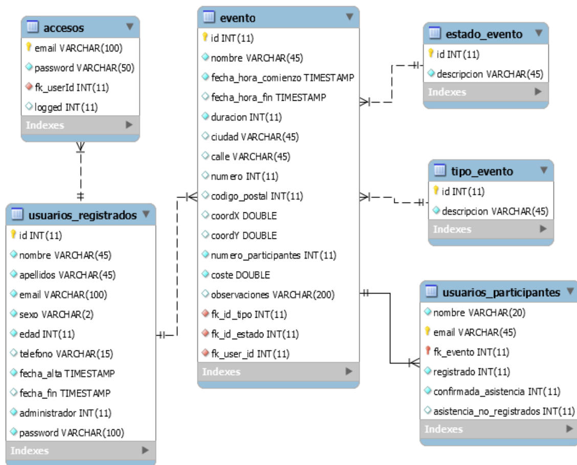
Figura 17. Modelo de base de datos.
