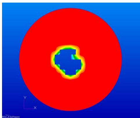
Figura 16. Área delaminada para un impacto de 2J .
