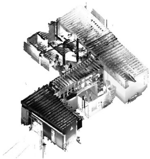
Levantamiento por escáner láser 3D y restitución fotogramétrica de la intervención de CUAC Arquitectura en San Jerónimo 17 (BIMdD, 2015).
