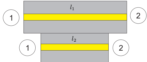
Fig. 1. Líneas microstrip para la caracterización de la permitividad de materiales de impresión 3D.
