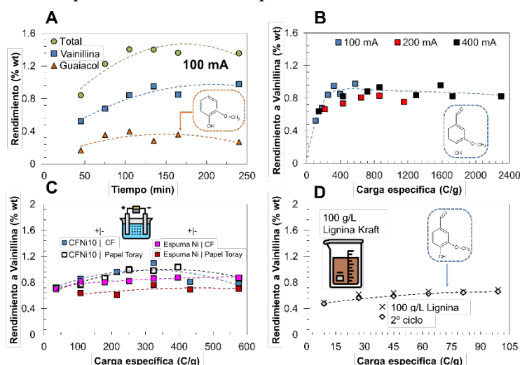
Figura 2 Rendimiento hacia vainillina, guaiacol y monómeros en la electrooxidación de una disolución de 25 g/L de lignina en función del tiempo de reacción a 100 mA (A). Rendimiento hacia vainillina en función de la carga específica a 100, 200 y 400 mA (B), empleando distintas configuraciones para los electrodos y 100 mA (C) y reutilizando el electrocatalizador CFNi10 a 100 mA y con 100 g/L de lignina (D).
