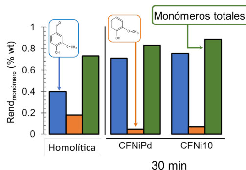
Figura 1. Rendimiento a vainillina, guaiacol y monómeros totales en la despolimerización electrooxidativa sin electrodo de trabajo y con CFNiPd y CFNi10 a 0.6 V vs SHE durante 30 min.
