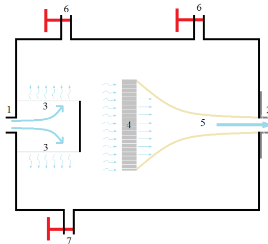
Figura 2.4. Detalle interior del depósito remansador.
