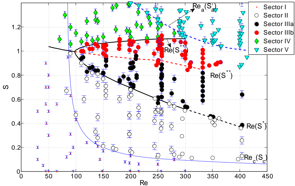
Figura 5.1. En el plano Re - S se representan los límites de régimen observados en el análisis teórico de estabilidad [Fernández-Feria y del Pino (2002)], las simulaciones numéricas [Sanmiguel-Rojas et al. (2008)] y los datos experimentales. Los datos experimentales corresponden a: sector I – Flujo estable (puntos rojos pequeños); sector II – Inestabilidades convectivas (puntos blancos); sector III – Inestabilidades en la expansión, que se corresponden con inestabilidades en la capa de cizalladura moviéndose aguas abajo (puntos negros) y Vórtices pulsantes en la capa límite (puntos rojos); sector IV – Rotura estable de vórtices (diamantes verdes); sector V – Rotura inestable de vórtices/Inestabilidades absolutas (triángulos azul turquesa). Predicciones teóricas [Fernández-Feria y del Pino (2002)] para la transición del régimen estable a convectivamente inestable [ Re_c(S_c) ], y de estado convectivamente inestable a absolutamente inestable [ Re_a(S_a) ] en un flujo de Hagen-Poiseuille con giro (líneas azul continuas y discontinuas, respectivamente). Predicción numérica [Sanmiguel-Rojas et al. (2008)] con línea negra continua desde las inestabilidades convectivas a las tridimensionales en la expansión [rama inferior, Re(S^*) ] y el inicio de la rotura estable de vórtice, rama superior, Re(S^{**}) . La línea gruesa discontinua es una transición experimental que extiende los resultados numéricos para números más altos de Reynolds [ Re(S^*) ] y la línea roja discontinua [ Re(S^{**}) ] es la transición experimental entre el sector IIIa y el sector IIIb.
