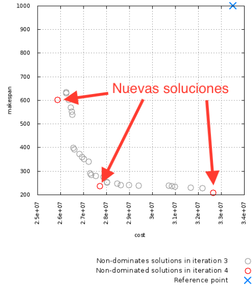
Fig. 6. Tercera iteración de iWASFGA en la instancia 8 employees and 64 tasks.
